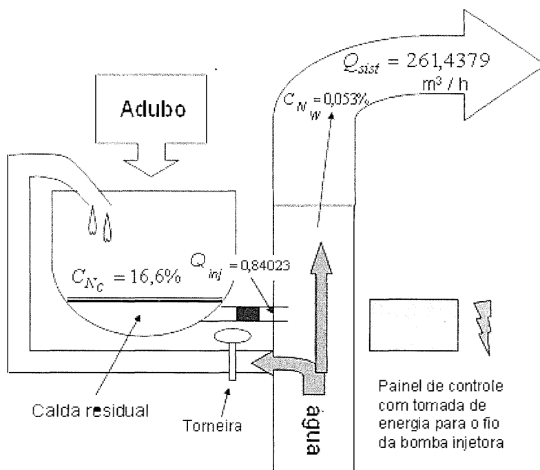
Figura 9 – Representação esquemática da injeção da calda fertilizante no pivô, bem como das vazões e das concentrações de nitrogênio na calda e na água de irrigação. É fundamental que haja uma calda residual no ato do reabastecimento, o que confere tempo hábil para esta operação
