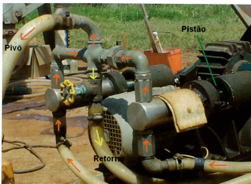
Figura 6 - Direções seguidas pela calda fertilizante: pivô e/ou retorno para o tanque
