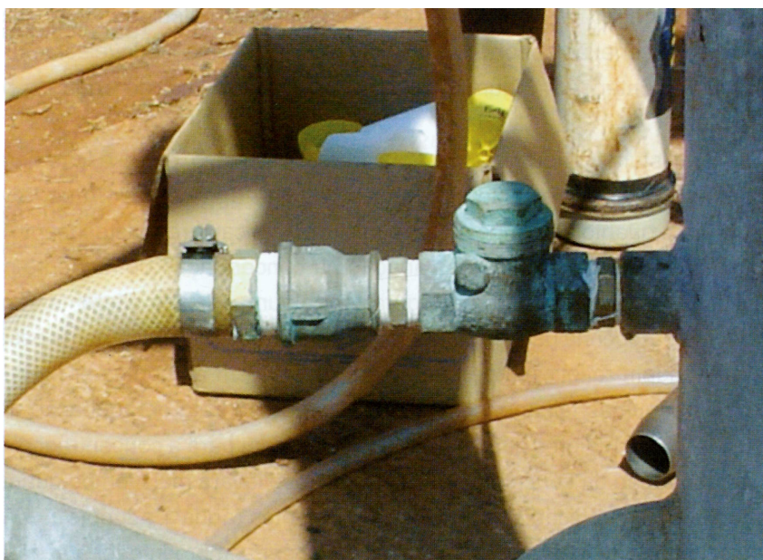
Figura 7 - Válvula de contenção: acima, um posicionamento equivocado da peça, que deveria trabalhar no sentido vertical, e acoplada a um cotovelo. Quando necessário, deve-se fazer a substituição da peça, que é constantemente submetida à ação corrosiva da calda fertilizante (muito mais concentrada que a água de irrigação contendo fertilizantes, que sai nos emissores)
