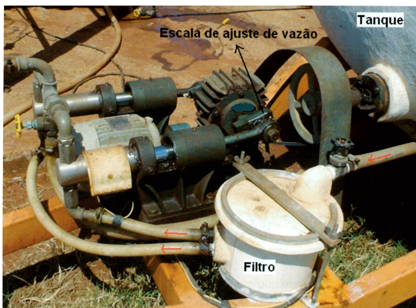
Figura 5 - Após deixar o tanque e antes de ser injetada, a calda fertilizante deve passar por um filtro, o qual deve ser constantemente limpo
