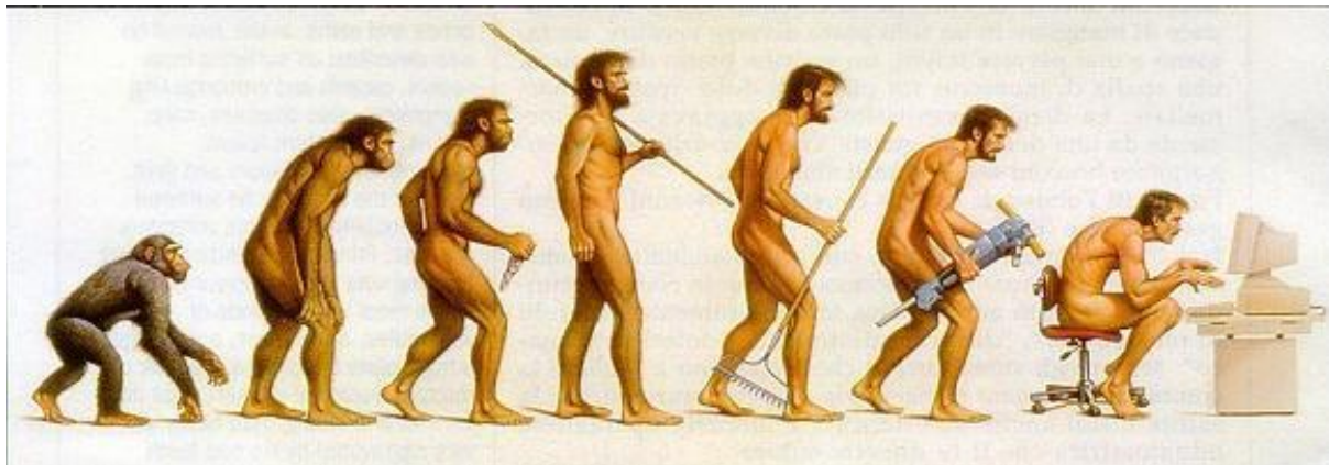
Evolution (?)
