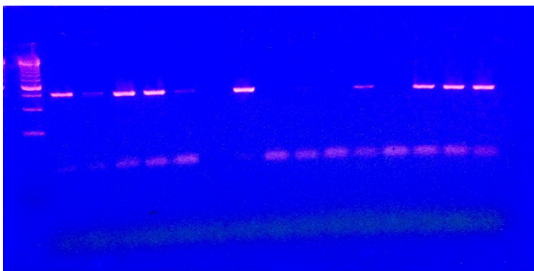
Figura 2 - Gel de agarose contendo amostras de DNA amplificado de L. monocytogenes oriundas de leite contaminado artificialmente para reação de PCR específico para Listeria monocytogenes
