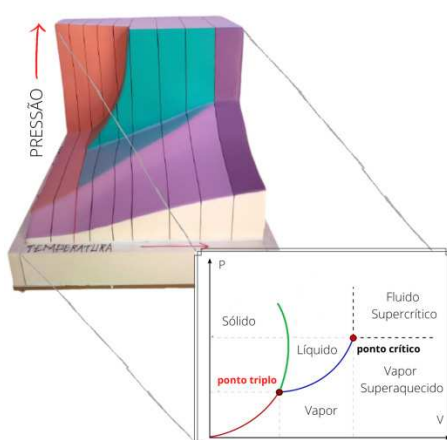
Figura 2d – Projeção do plano “Pressão x Temperatura”
