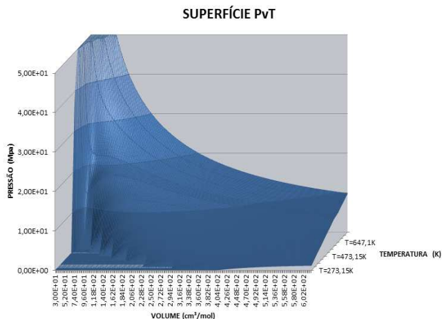
Figura 6 – Simulação da superfície a partir do equilíbrio líquido - vapor
