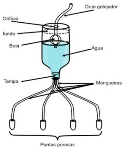
Figura 2. Irrigador solar evidenciando-se as partes principais.
