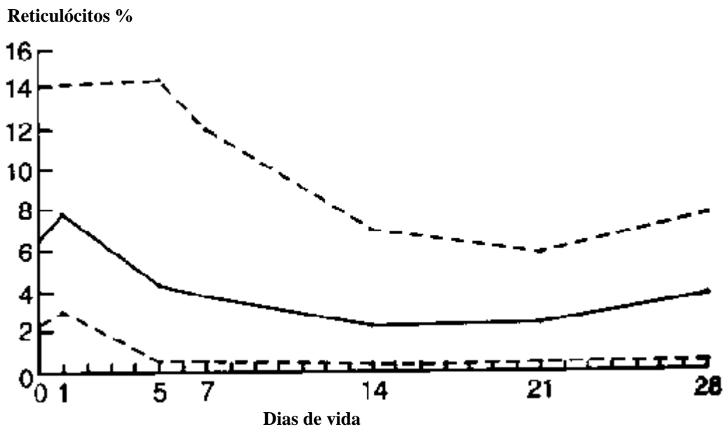
3.4 - Média \pm 2 desvios-padrão dos valores de reticulócitos no RN pré-termo (<36semanas)
