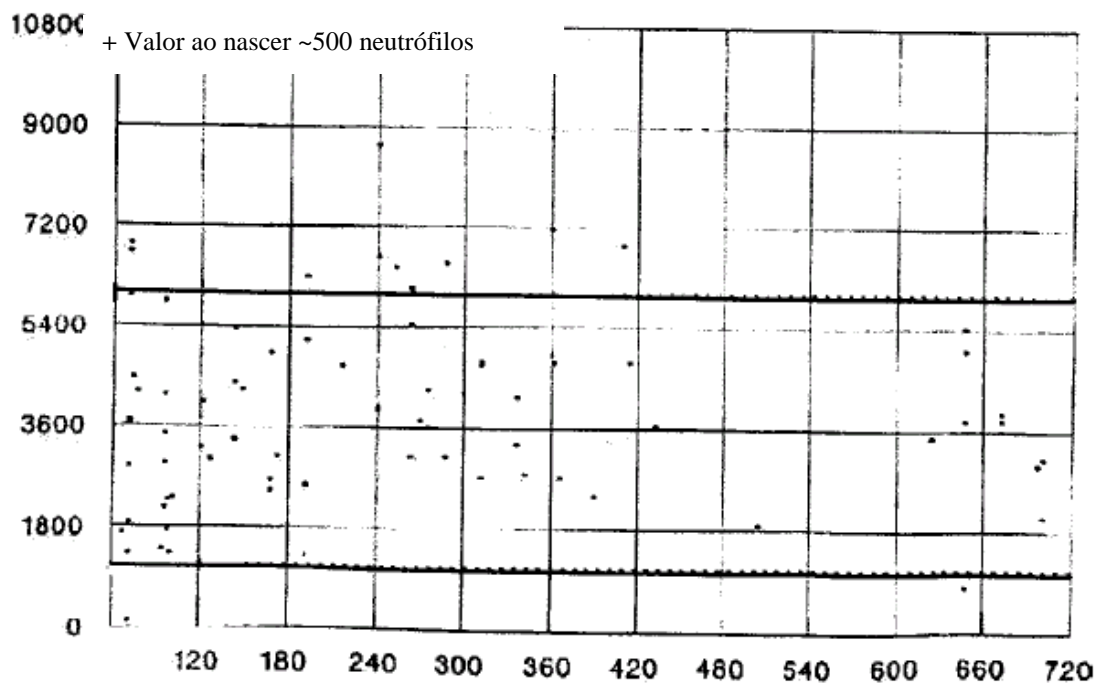
7. Número de Neutrófilos totais para RN MBP segundo o tempo de vida (Mouzinho)
