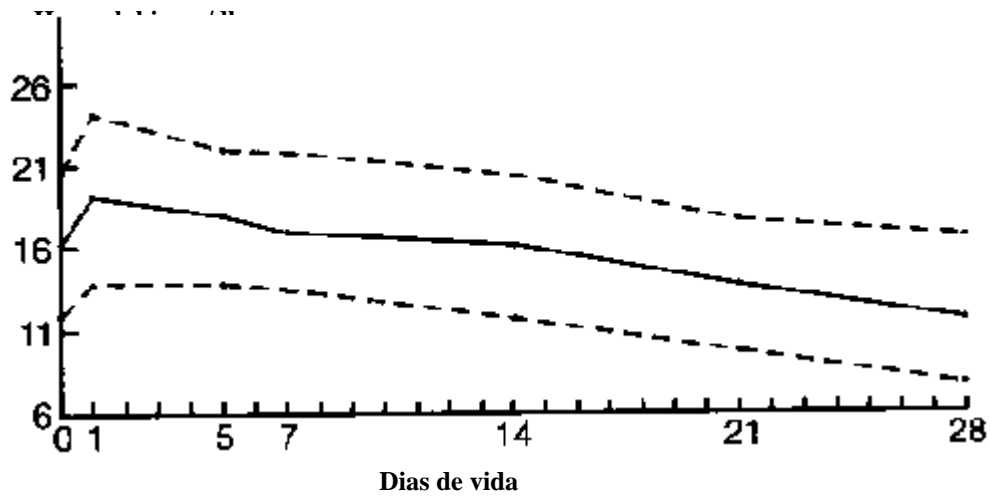
3.3 - Média \pm 2 desvios-padrão dos valores de hemoglobina no RN pré-termo (<36semanas)
